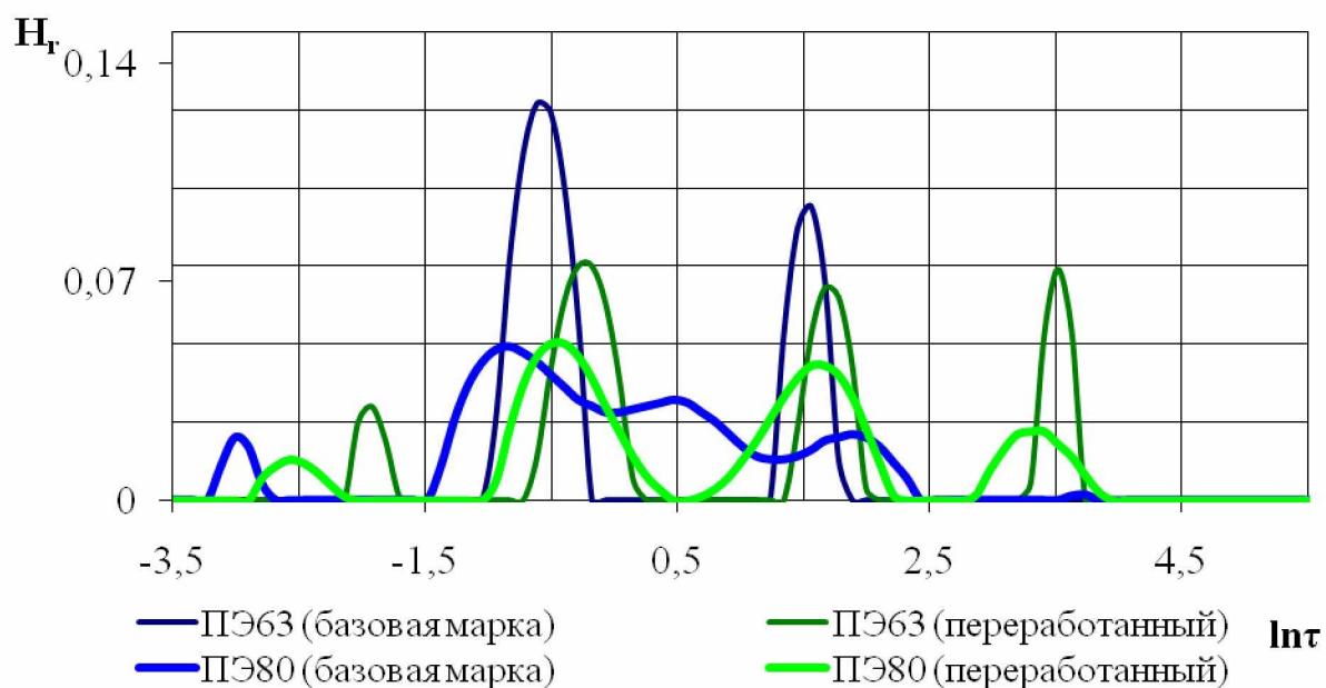
Рис. 3 Изменения спектров времён релаксации давления ПЭ 63 и ПЭ 80 в результате термомеханодеструкции.
