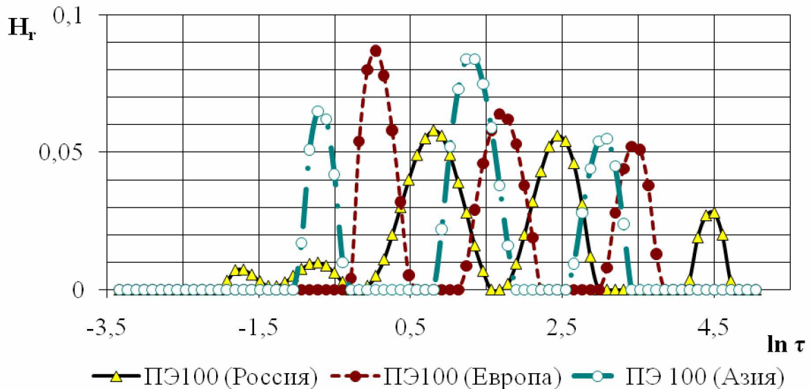
Рис. 4 Спектры времён релаксации давления ПЭ 100 различных производителей а – спектры, рассчитанные по аппроксимационной методике (по формуле Шварцеля –Ставермена); б – спектры, рассчитанные по регуляризационной методике.
