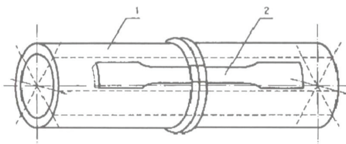
Рисунок 2 – Схема вырезки образцов из сварного соединения для испытания на осевое растяжение
