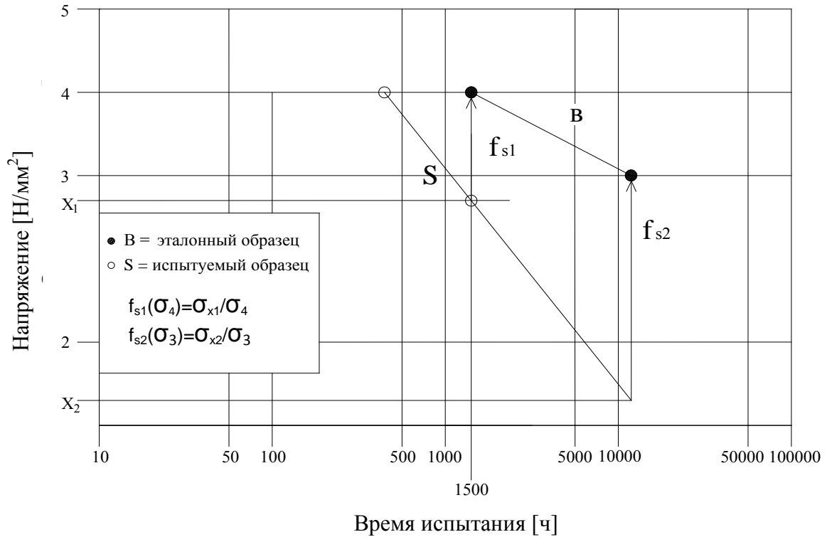
Рисунок 7 – Схема определения коэффициента прочности сварного шва f_s при длительных испытаниях на ползучесть при растяжении
