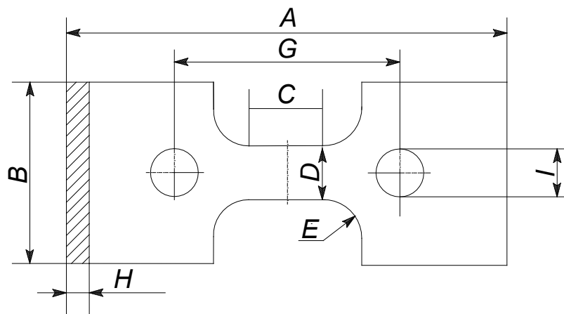
Рисунок 4 – Испытуемый образец, тип 3
