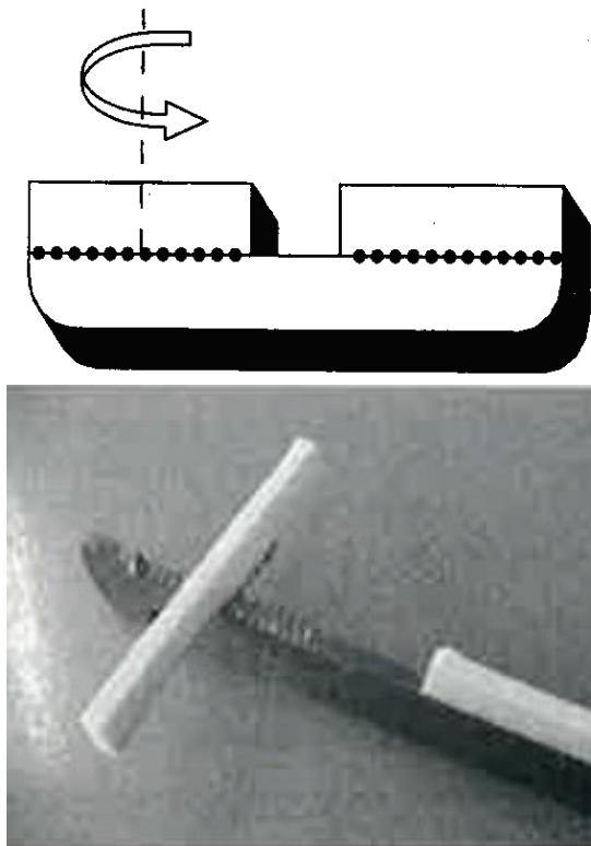
Рисунок Б 4 – Сдвиг кручением вручную
