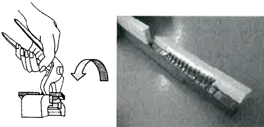
Рисунок Б 6 – Испытание на радиальное расслаивание (RPT) для соединений, выполненных сваркой с закладными нагревателями (ЗН) и нагретым инструментом (НИ) в раструб
