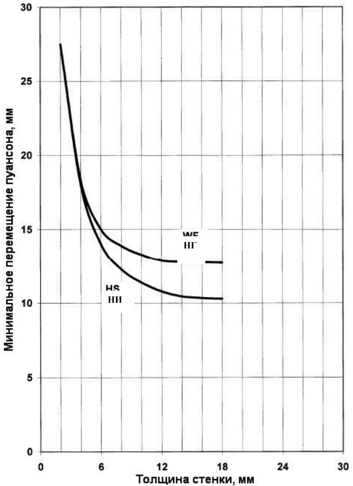
Рисунок В 10 – Минимальное перемещение пуансона для ПВДФ в зависимости от толщины для разных методов сварки. Нижняя кривая – для сварки нагретым инструментом встык, верхняя – для прутковой сварки нагретым газом
