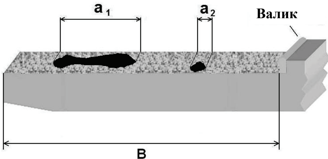
Рисунок А 2 – Оценочная длина ( B ) и примеры дефектов ( a_1 и a_2 ) в случае образцов, которые выполнены сваркой нагретым инструментом (НИ) в раструб
