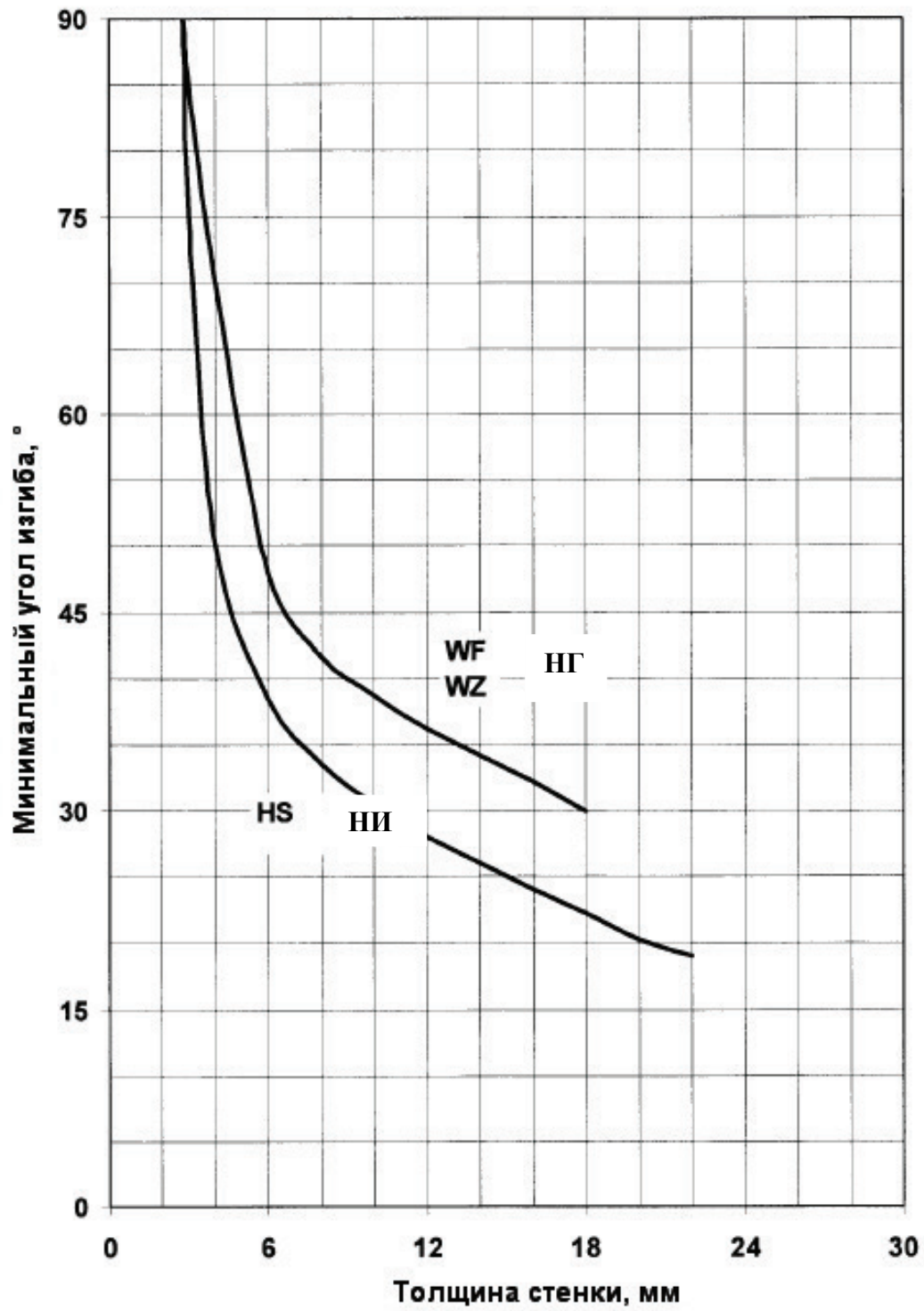
Рисунок В 4 – Минимальный угол изгиба для ПВДФ в зависимости от толщины для разных методов сварки. Нижняя кривая – для сварки нагретым инструментом встык, верхняя – для прутковой сварки нагретым газом
