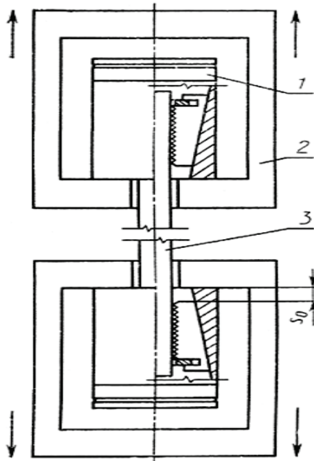
1 – зажим; 2 – приспособление для испытания; 3 – образец
