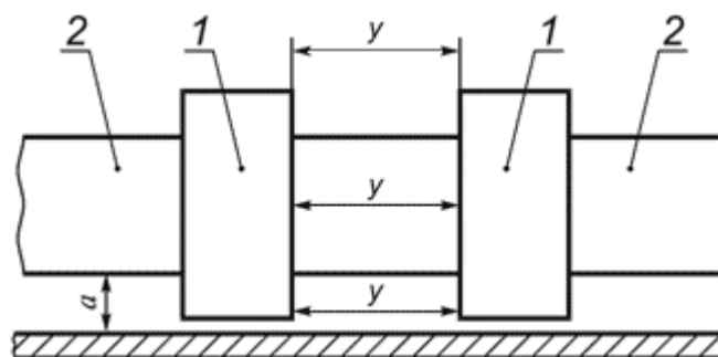
б) Трубы сведены (замер y )
