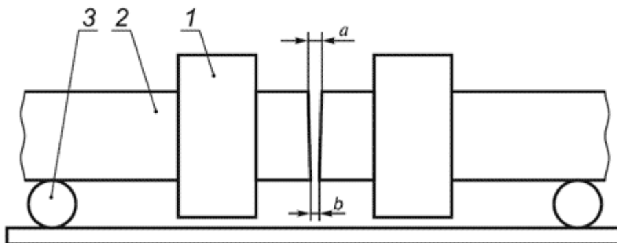
а) Поддерживающие цилиндры присутствуют
