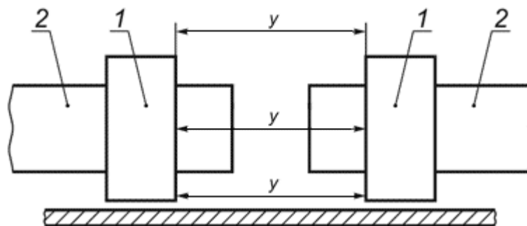
с) Зажимы разведены (замер y ) 1 - зажим; 2 - труба; a - не менее 200 мм в низшей точке
